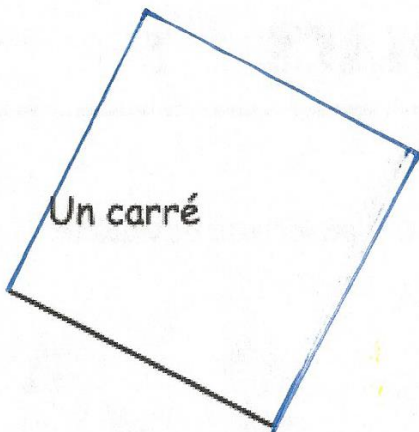
Un parallélogramme
