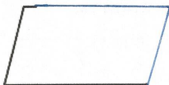
Un parallélogramme
